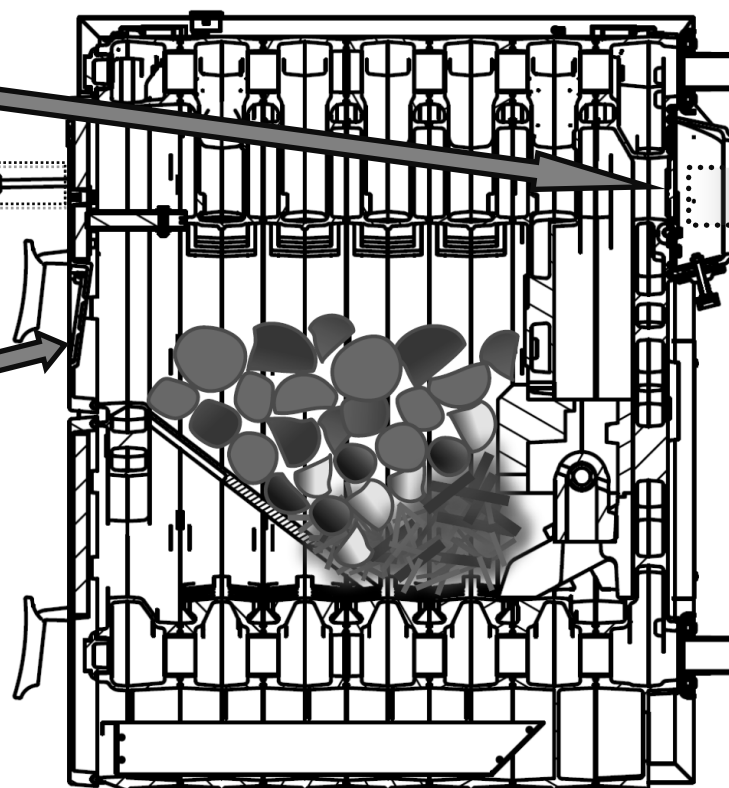
Obr. č. 25 Nastavení kotle pro měření emisí
