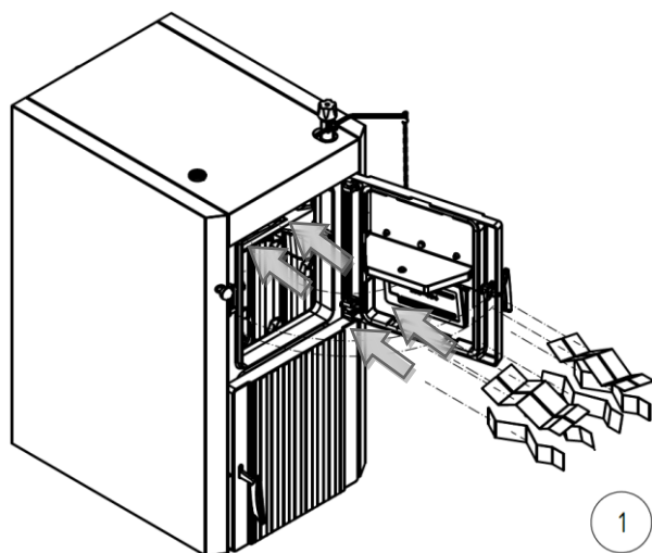
Obr. č. 26 Umístění turbulátorů v kotli
