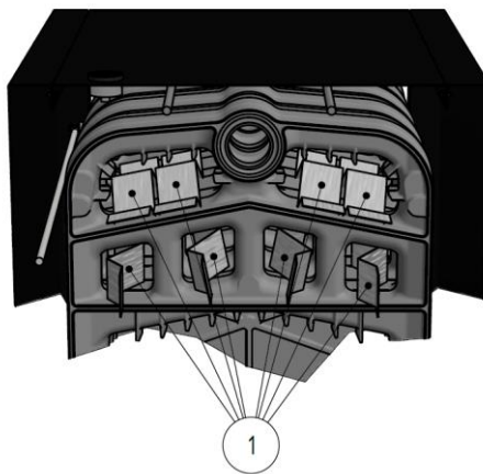
1. Turbulátory dle velikosti kotle
