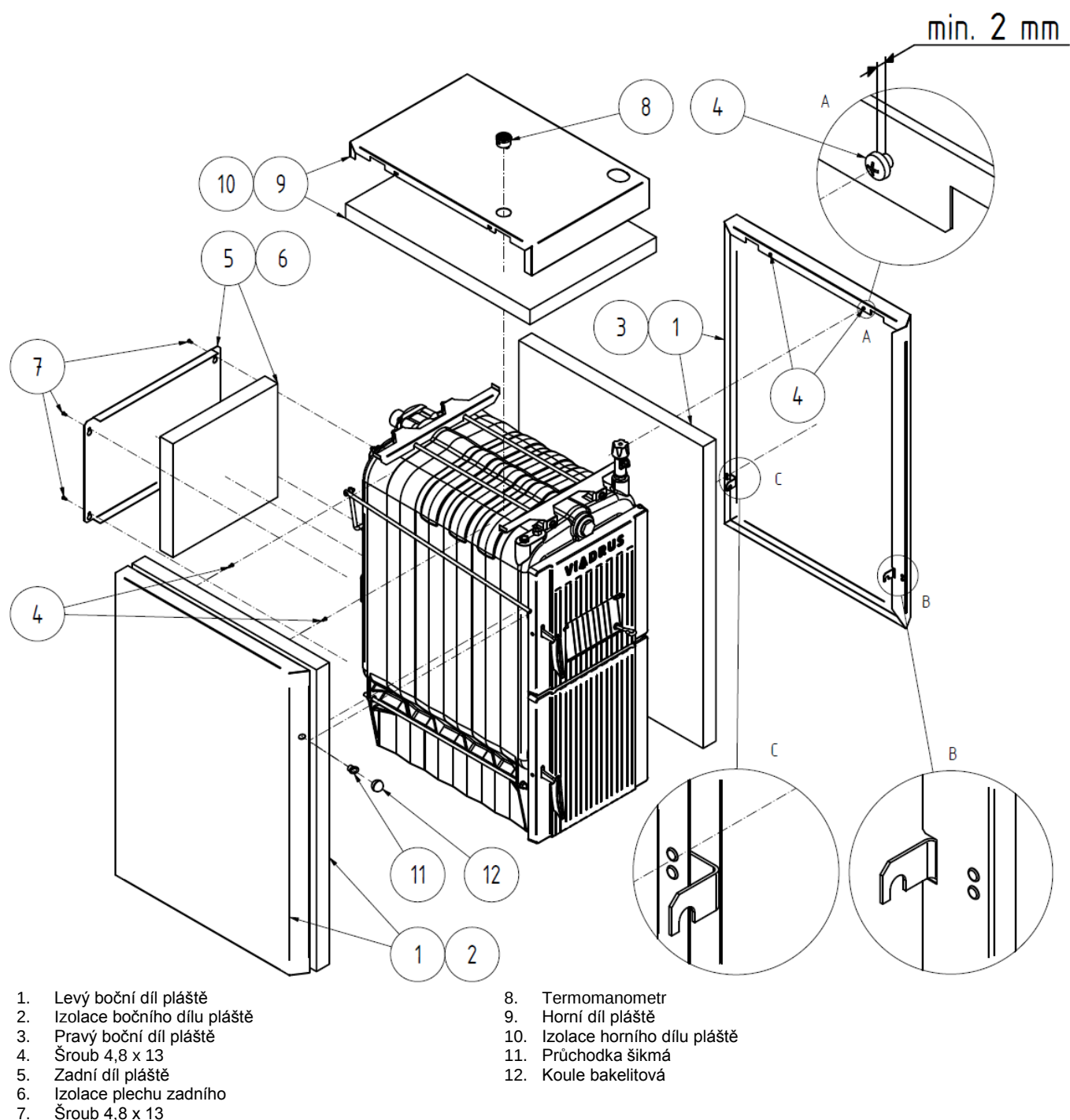
Obr. č. 18 Montáž bočních dílů pláště
